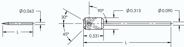
T (TUNGSTEN P/N: 635-063-SERIES)
