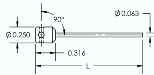
H-90 (TUNGSTEN HOLDER ASSEMBLY 90 DEG P/N: 002-0771)
